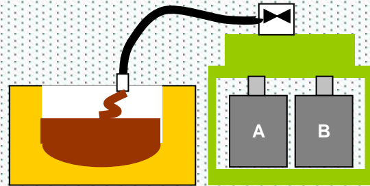
2. Vergießen der Form durch RAMPF Tooling
